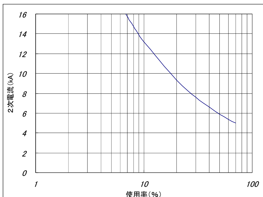
使用率曲線
