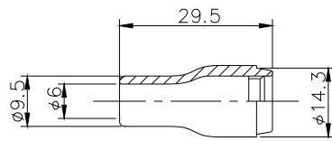
セラミックノズル : 13N08
