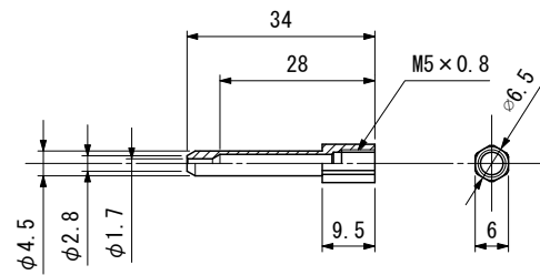
コレットチャック : MB0312181
