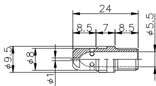
コレットボディ : MB0312174-10
