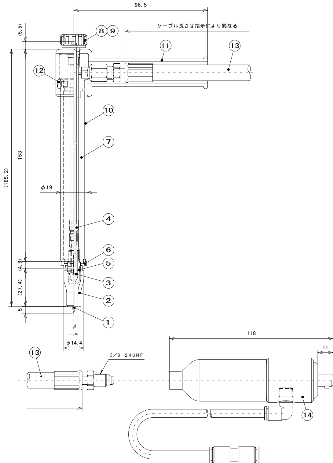
① 外形図 (単位: mm)
