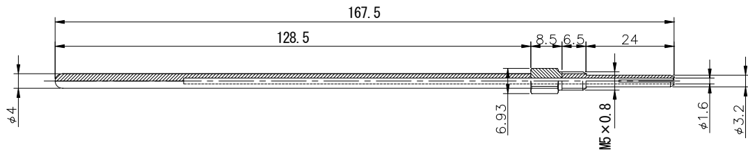
コレットボディ : MB0312174-10
