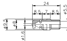
コレットボディ : MB0312174-16
