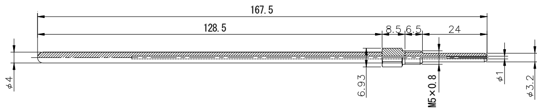
コレット : MB0312182-16
